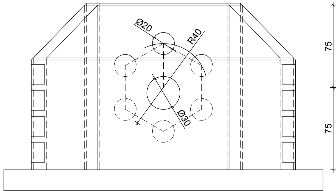
Seitenansicht M 1:2
