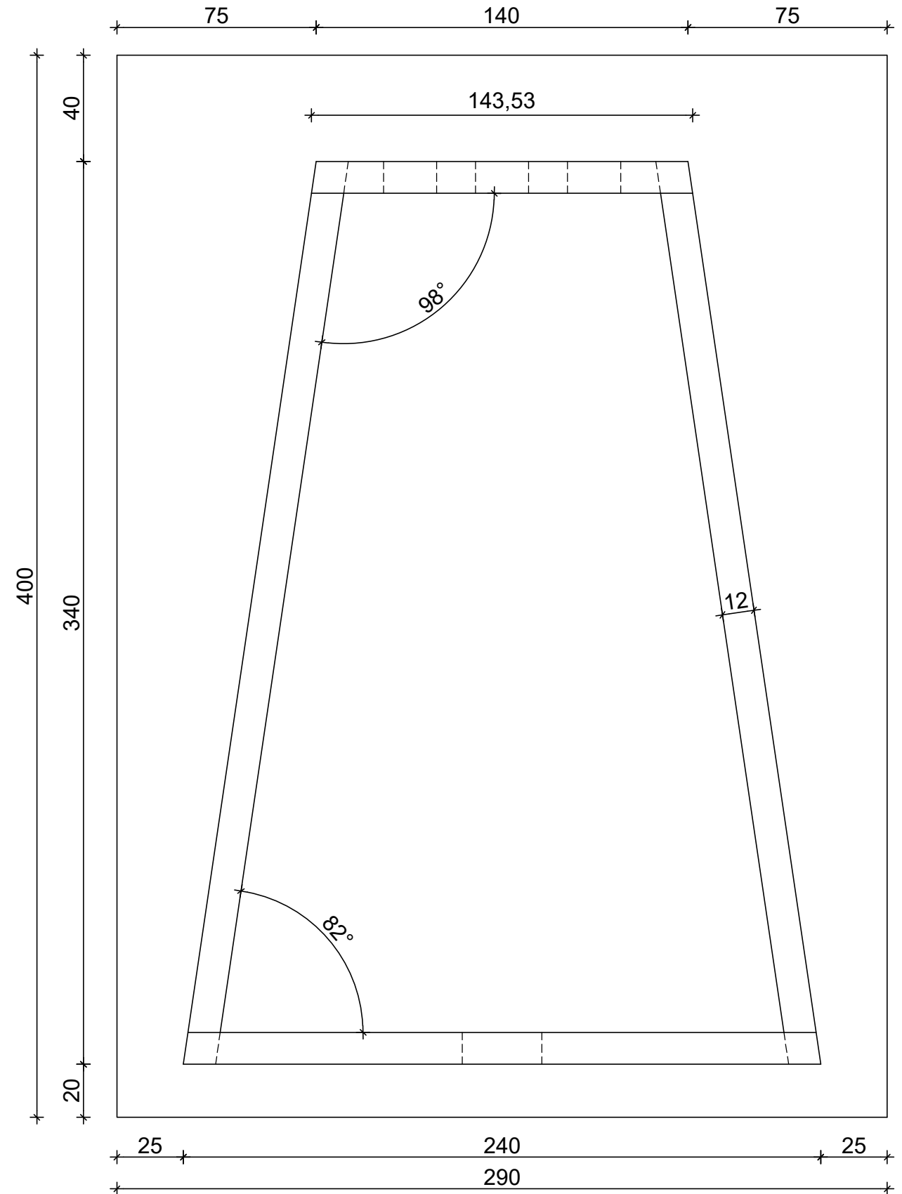
Grundriss M 1:2
