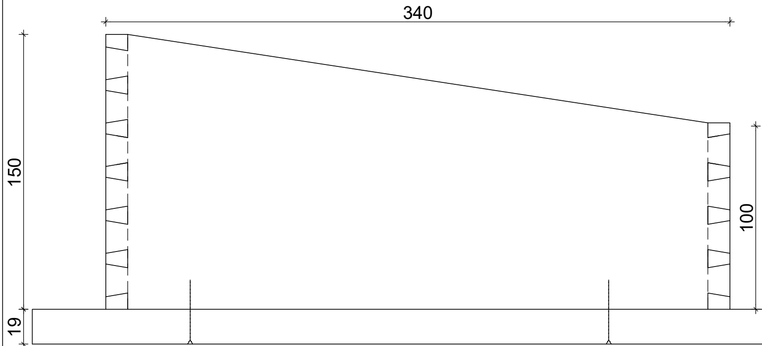
Seitenansicht M 1:2
