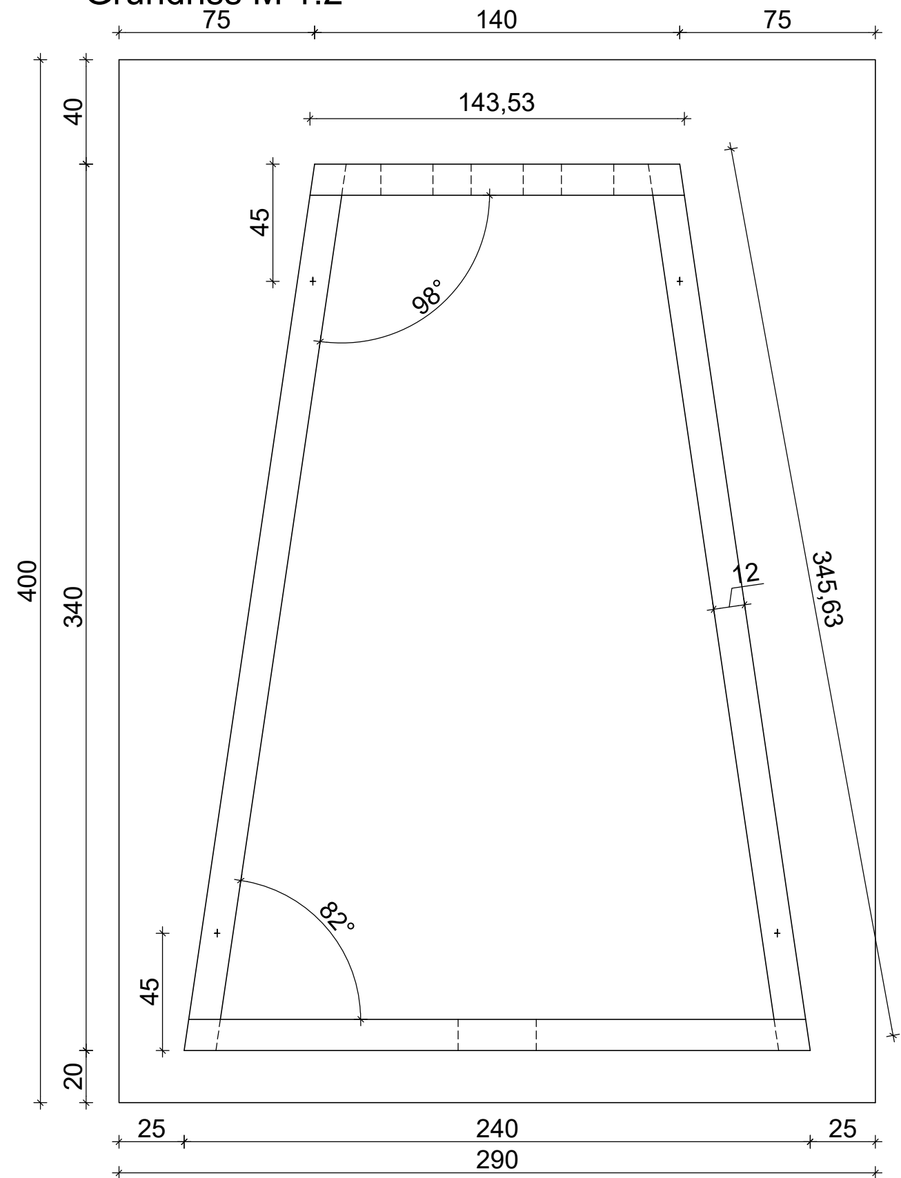
Grundriss M 1:2
